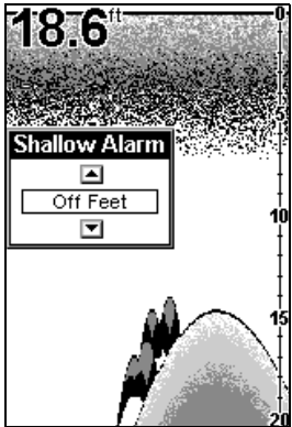
Shallow Alarm menu.
